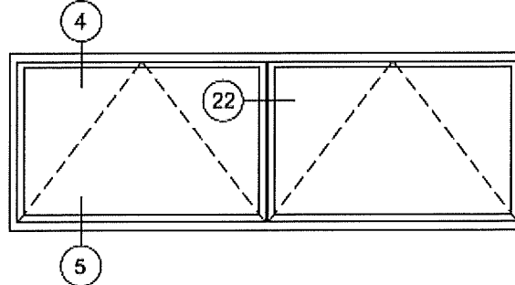
DOUBLE AWNING
